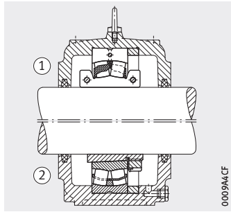
Festlager S30
