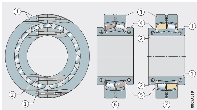
Bild 8 Innenkonstruktion der Lager mit integrierten Spannringen
