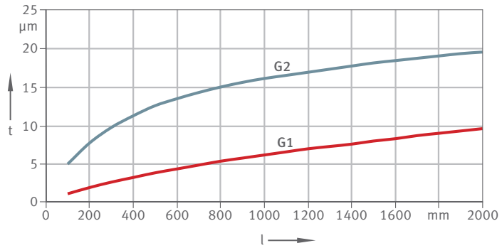
22 Genauigkeitsklassen und Parallelitätstoleranzen der Führungsschienen
