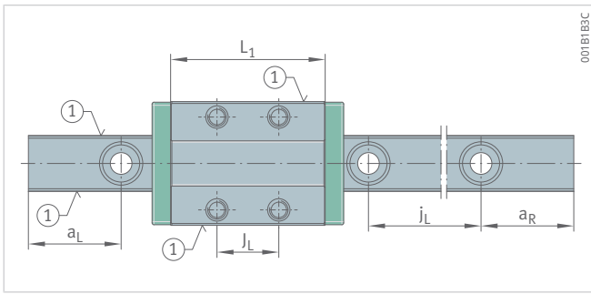
KUEM..-E, Ansicht um 90° gedreht
