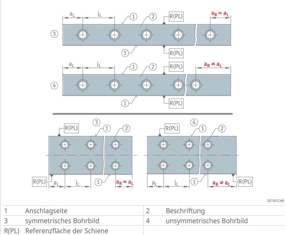
☞18 Bohrbilder bei Führungsschienen mit 1 oder 2 Bohrungsreihen
