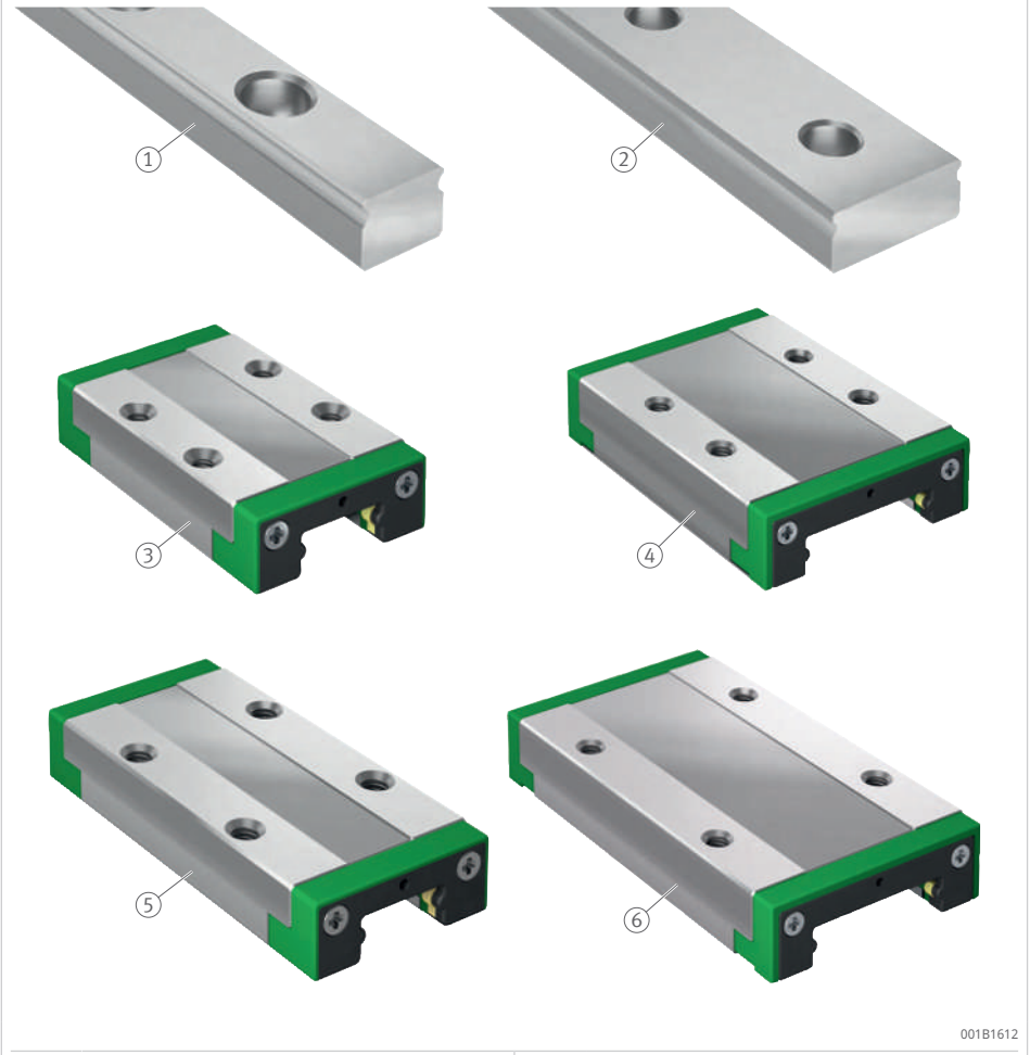
17 Produktübersicht, Führungsschienen und Führungswagen mit Schmierstoff-Reservoir
