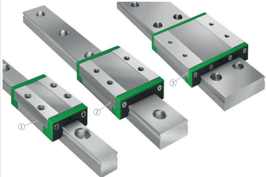
☞16 Produktübersicht, Kugelumlaufsystem bestehend aus Führungswagen und Führungsschiene
