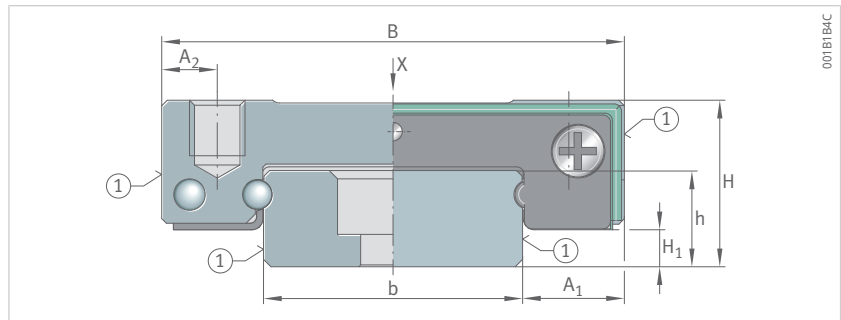
KUEM...-E-W
