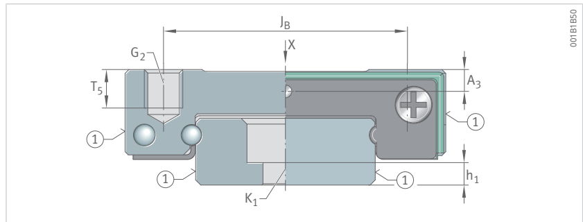
KUEM..-E-W (Baugröße 07, 09, 12)
