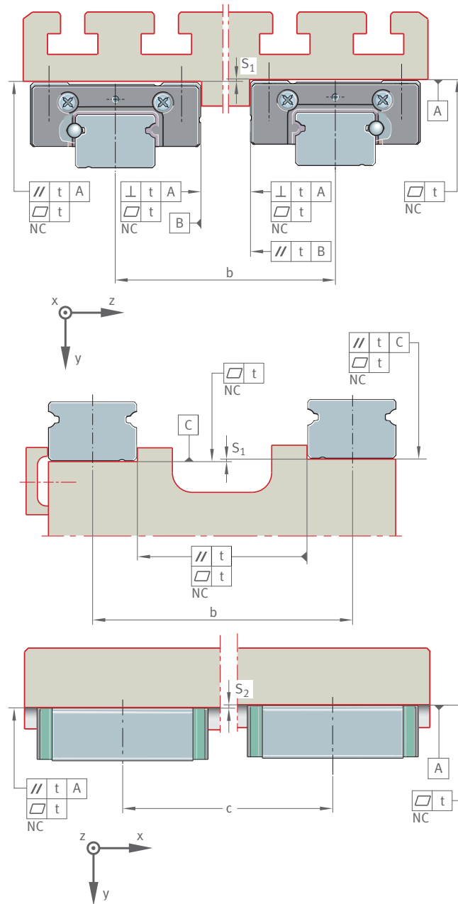
31 Toleranz der Anschlussflächen und Parallelität der montierten Führungsschienen und Führungswagen
