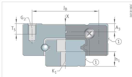
KWEM05 mit TKDM05
