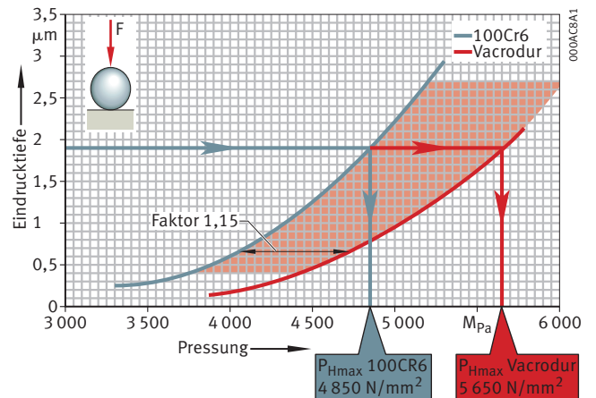
Bild 5: Eindringtiefe in Abhängigkeit zur Drückung
