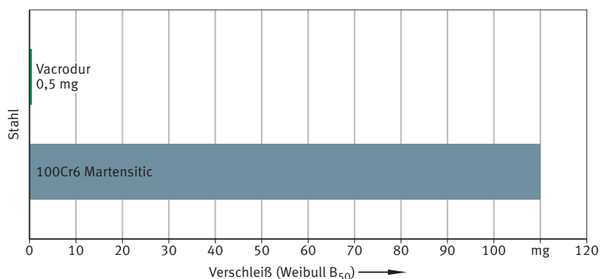
Bild 7: Verschleißbeständigkeit im Vergleich
