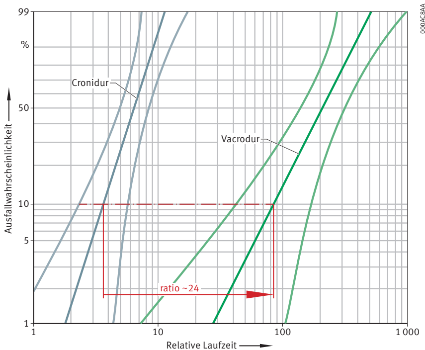
Bild 6: Lebensdauer unter Kontamination
