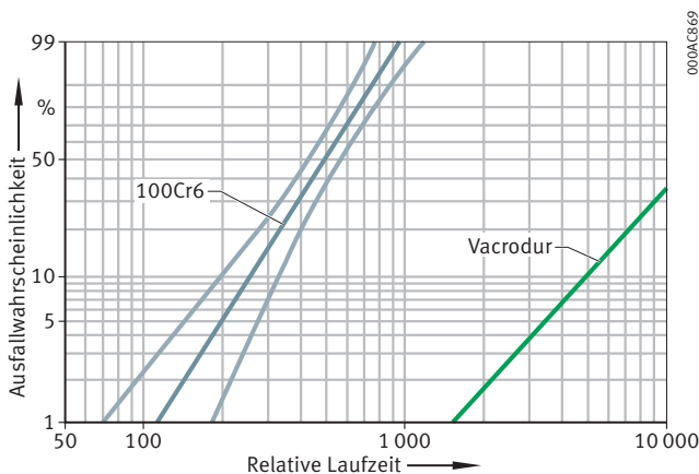
Bild 4: Lebensdauer unter Mischreibung
