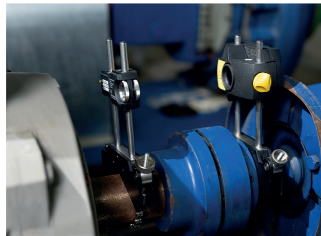
Outils industriels – Alignement Industrie : LASER-EQUILIGN2 assure toujours un alignement correct de vos machines grâce à la technologie de laser unique
