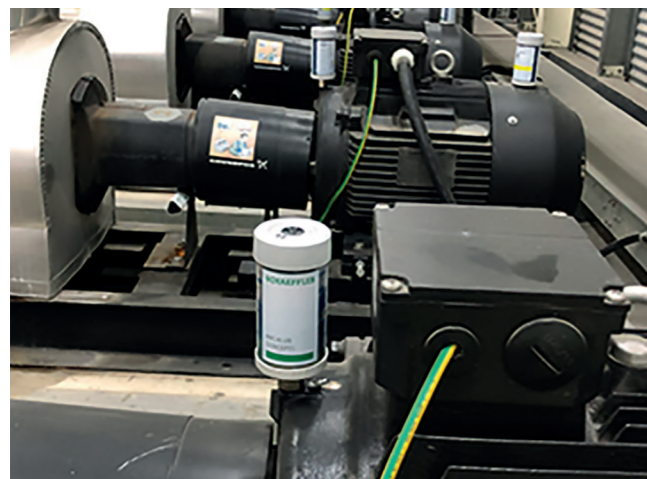
Solution de lubrification Industrie : CONCEPT1 lubrifie des dizaines de moteurs
