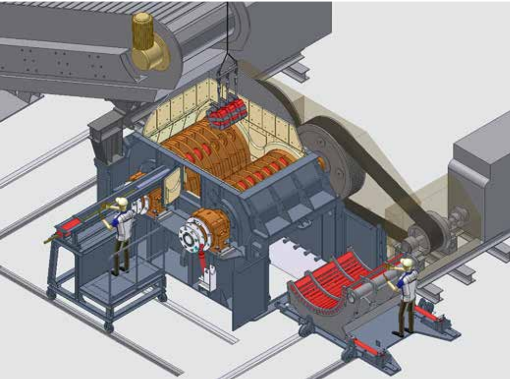
锤式破碎机
