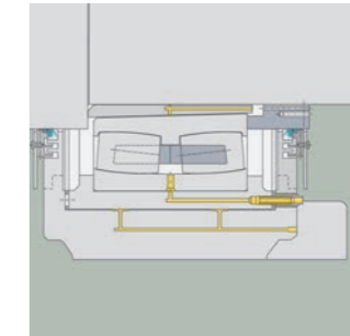
Corps de palier à manchon coulissant
