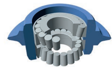
Calcul du roulement d'un disque de découpe avec le programme de calcul Bearinx de Schaeffler
