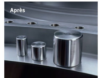
Piste de roulement rectifiée, nouveaux rouleaux avec serrage adapté
