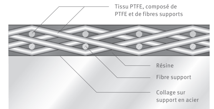
Composition du revêtement ELGOGLIDE
