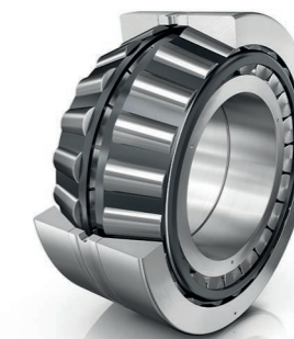
2-reihiges Kegelrollenlager in X-Anordnung
