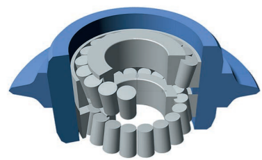
Berechnung einer Schneidenlagerung mit dem Schaeffler-Berechnungsprogramm Bearinx
