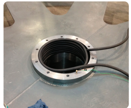
Erwärmung einer Bohrung zur Montage von Lager oder Achse
