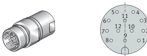
46 Connettore interfaccia SIN COS 1Vss + REF
