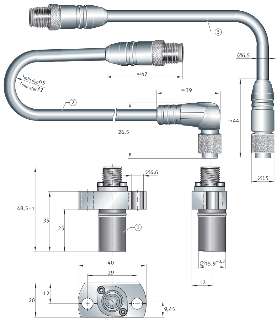
68 Dimensioni cavo di collegamento e sonda
