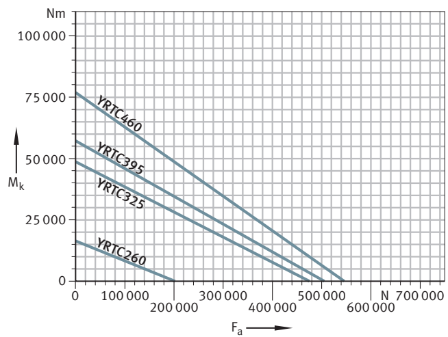
21 Diagramma statico dei carichi limite per YRTC260 - YRTC460
