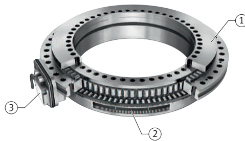
37 Sistema di misurazione induttivo integrato nel cuscinetto, incrementale
