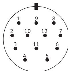
67 Piedinatura dei connettori a flangia a 12 poli
