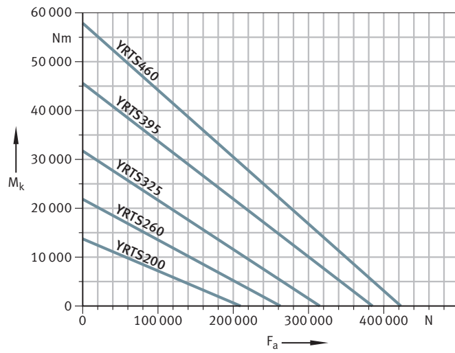
24 Diagramma statico dei carichi limite per YRTS200 - YRTS460
