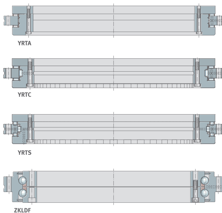
1 Cuscinetti assiali-radiali e cuscinetti assiali a sfere a contatto obliquo di Schaeffler
