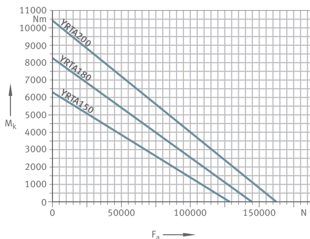
17 Diagramma statico dei carichi limite per YRTA150 - YRTA200
