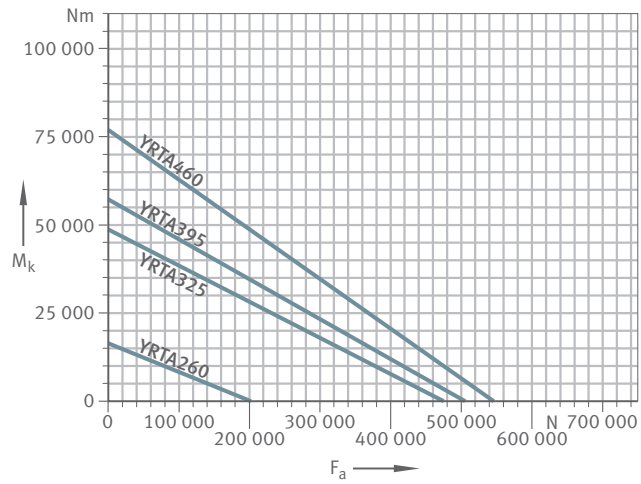
18 Diagramma statico dei carichi limite per YRTA260 - YRTA460
