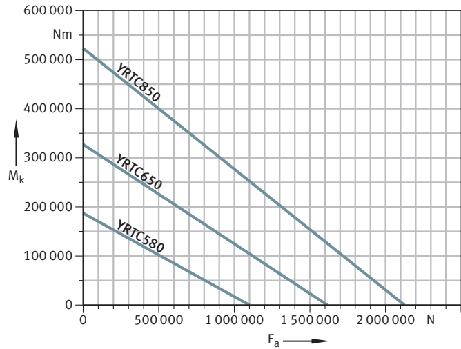
22 Diagramma statico dei carichi limite per YRTC580 - YRTC850
