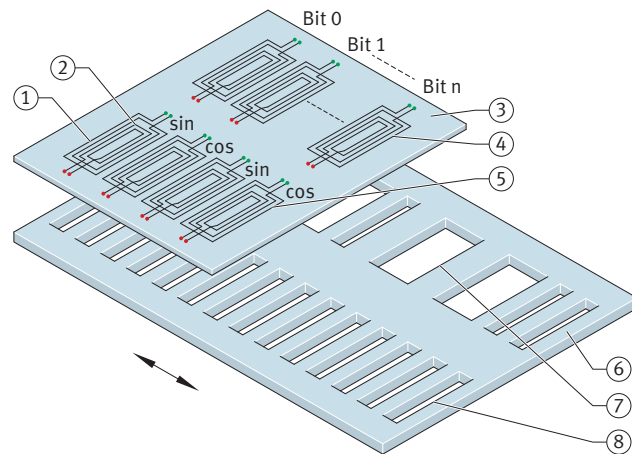
41 Principio di funzionamento dei sistemi di misurazione angolare induttivi assoluti AMOSIN®
