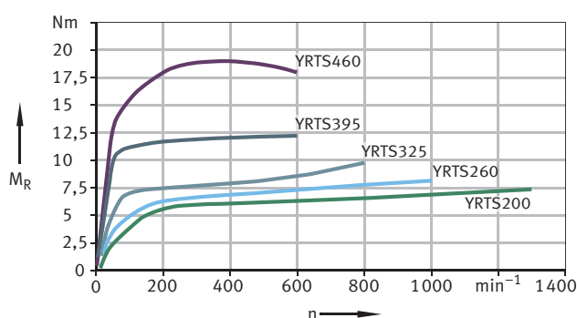
28 Momenti di attrito come valori indicativi per YRTS, valori determinati statisticamente da serie di misurazioni
