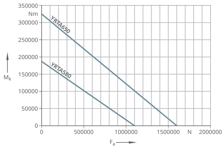
19 Diagramma statico dei carichi limite per YRTA580 - YRTA650
