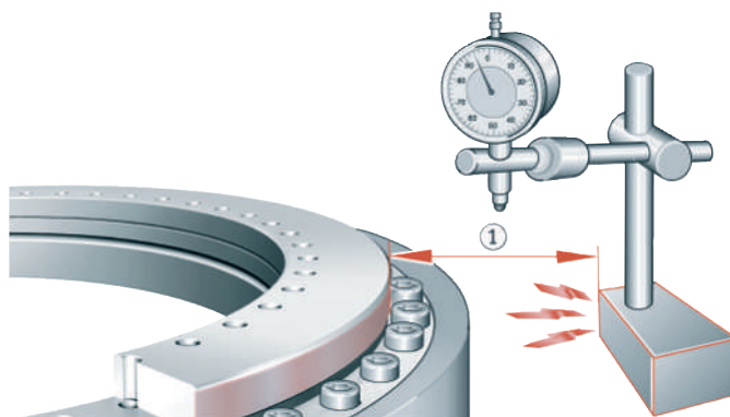
63 Distanza minima tra il supporto magnetico per misuratore e il disco ondolato
