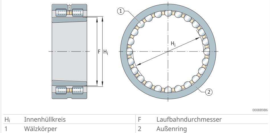
44 Innenhüllkreis bei Zylinderrollenlagern NNU49SK
