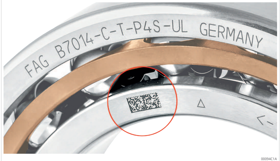
37 DataMatrix-Code auf Wälzlager
