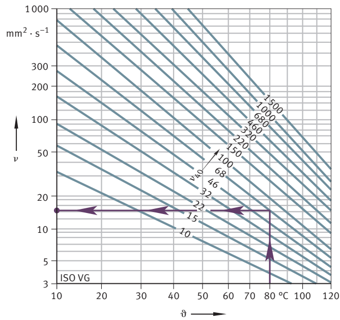
16 V-/T-Diagramm
