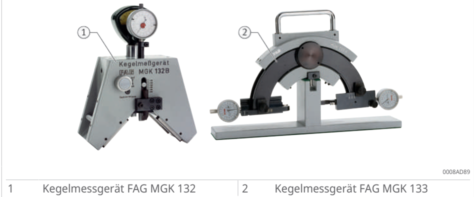
43 Kegelmessgeräte
