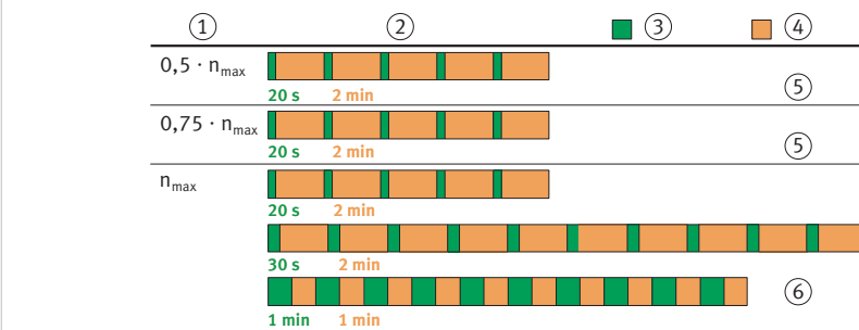
18 Fettverteilungslauf von offenen und abgedichteten Spindellagern
