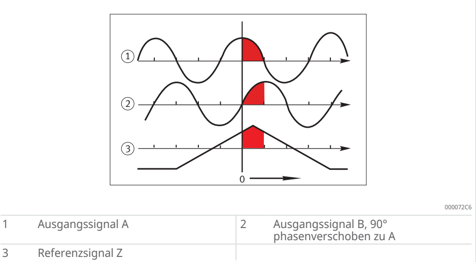
66 Referenzsignalposition
