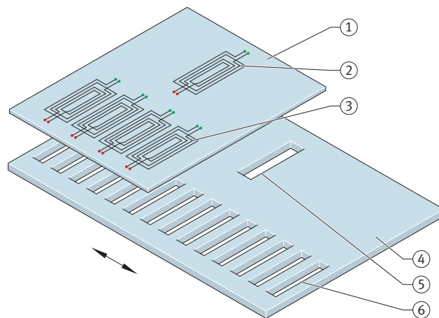
42 Wirkprinzip von induktiven, inkrementellen AMOSIN® Winkelmesssystemen
