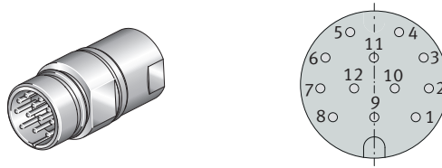
46 Steckverbinder Schnittstelle SIN COS 1Vss + REF
