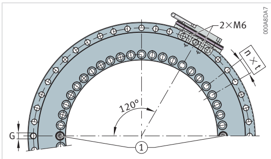
Bohrungsbild, radial anschraubarer Messkopf
