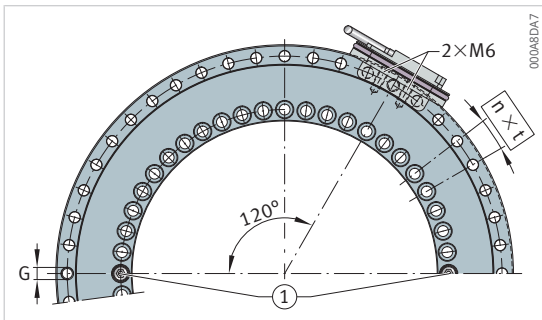
Bohrungsbild, radial anschraubbarer Messkopf
