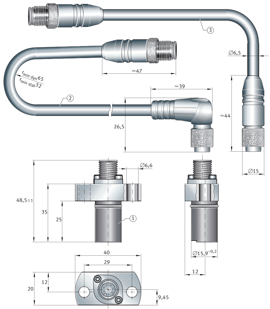
68 Abmessungen Verbindungskabel und Messkopf
