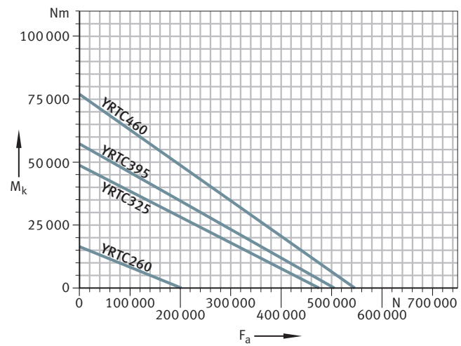
21 Statisches Grenzlastdiagramm für YRTC260 bis YRTC460
