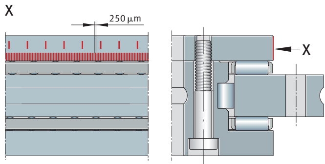
56 Maßverkörperung
