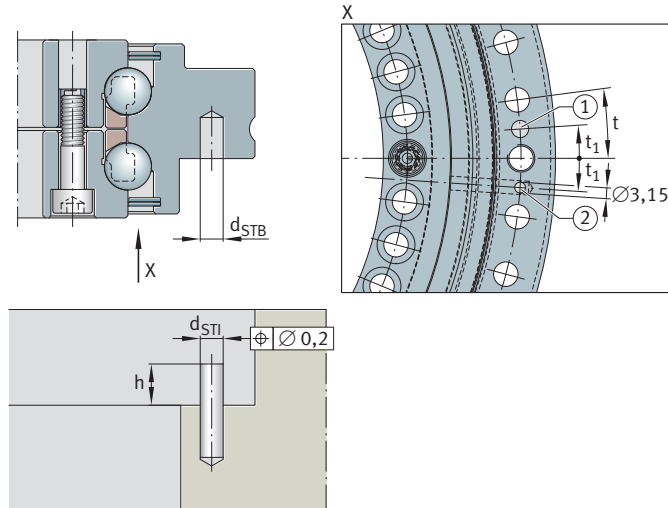
34 Montageerleichterung bei axialer Schmierbohrung
