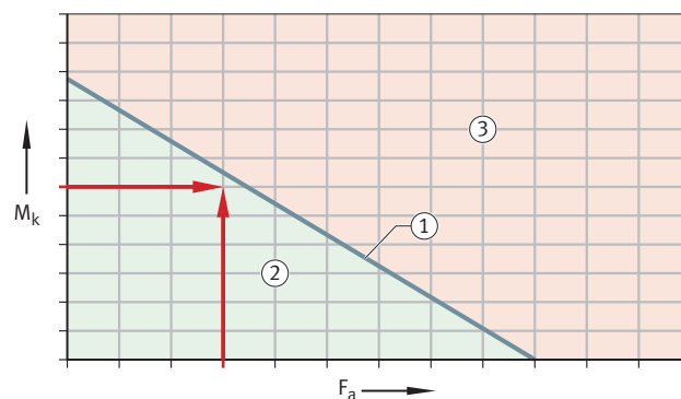
16 Beispiel für statisches Grenzlastdiagramm
