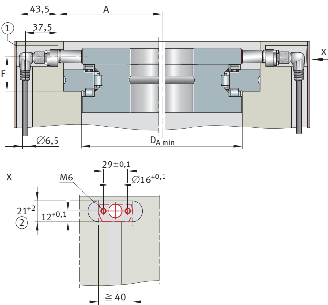
72 Gestaltung Anschlusskonstruktion und diametrale Anordnung der Messköpfe
