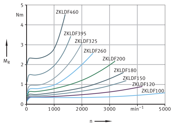
29 Reibmomente als Richtwerte für ZKLDF, statistisch ermittelte Werte aus Messreihen
