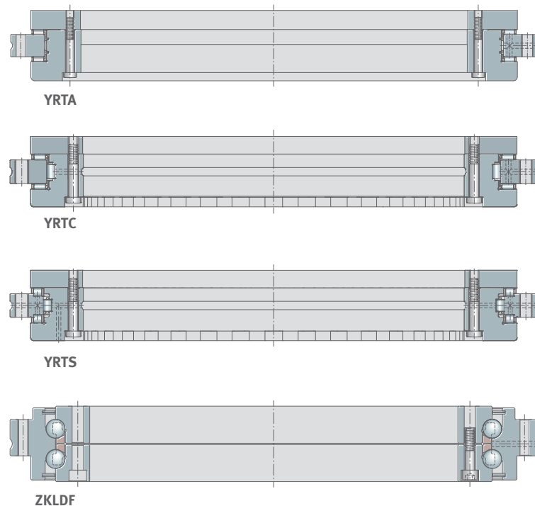
1 Axial-Radiallager und Axial-Schräggugellager von Schaeffler
