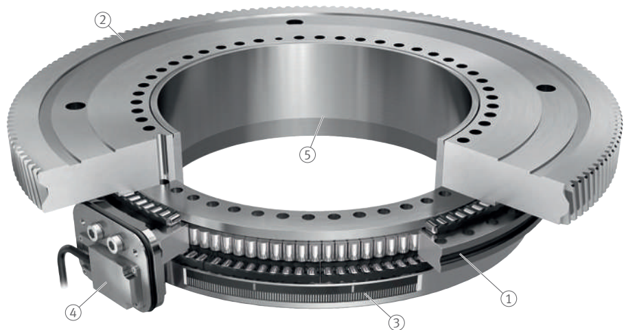
77 Axial-Radiallager YRTCGMA mit schrägverzahnter Wellenscheibe und induktiven Messsystem
