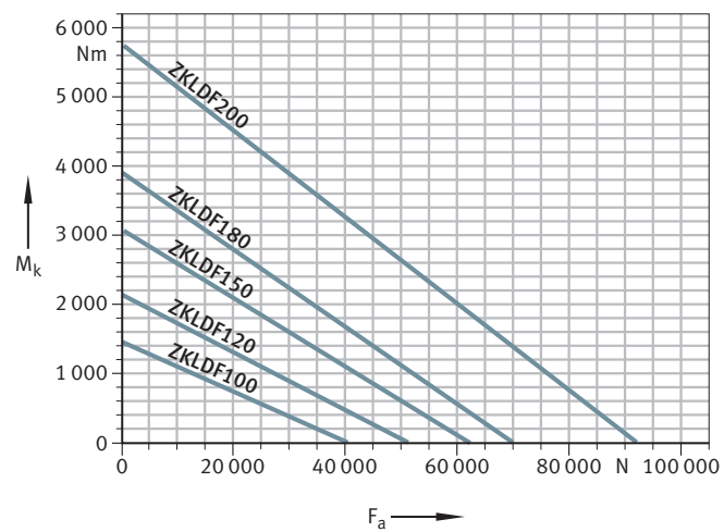
26 Statisches Grenzlastdiagramm für ZKLDF100 bis ZKLDF200
