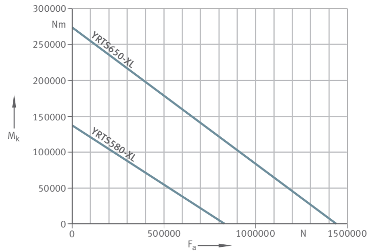
25 Statisches Grenzlastdiagramm für YRTS580-XL und YRTS650-XL
