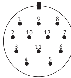
67 Steckerbelegung Flanschstecker 12-polig
