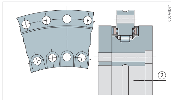
Schaubild bei YRTS325
