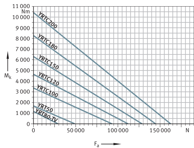
20 Statisches Grenzlastdiagramm für YRT50 bis YRTC200
