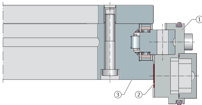
38 Absolutwert Winkelmesssystem
