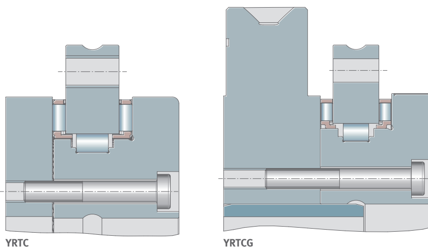
76 Weiterentwicklung der Lagerkonstruktion von YRTC zu YRTCG
