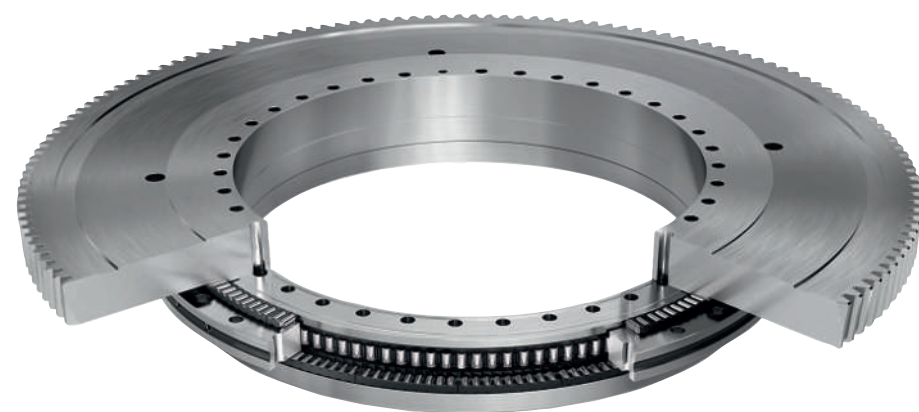
75 Axial-Radiallager YRTCG mit schrägverzahnter Wellenscheibe
