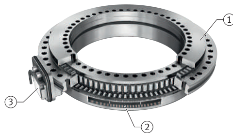
37 Lagerintegriertes induktives Messsystem, inkrementell
