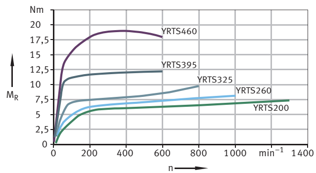
28 Reibmomente als Richtwerte für YRTS, statistisch ermittelte Werte aus Messreihen
