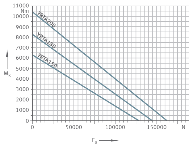
17 Statisches Grenzlastdiagramm für YRTA150 bis YRTA200
