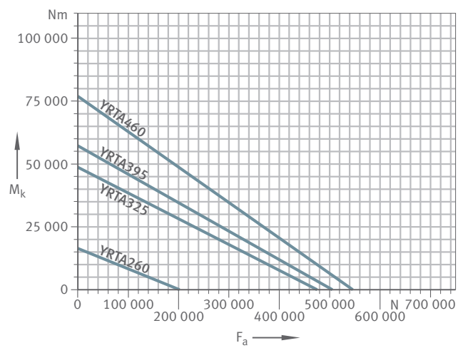
18 Statisches Grenzlastdiagramm für YRTA260 bis YRTA460
