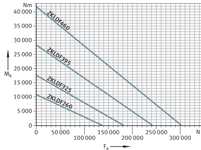
27 Statisches Grenzlastdiagramm für ZKLDF260 bis ZKLDF460
