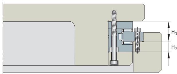
31 Anschlussmaß H 1 , H 2
