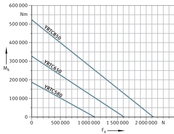
22 Statisches Grenzlastdiagramm für YRTC580 bis YRTC850
