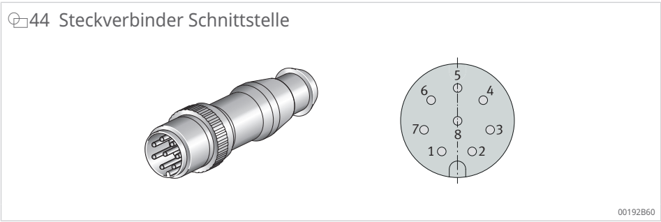
25 Anschlussbelegung
