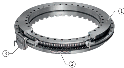
36 Lagerintegriertes induktives Messsystem, absolut
