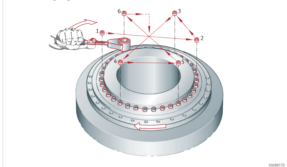
35 Befestigungsschrauben anziehen
