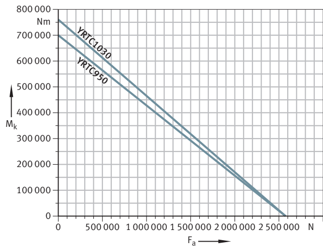
23 Statisches Grenzlastdiagramm für YRTC950 bis YRTC1030
