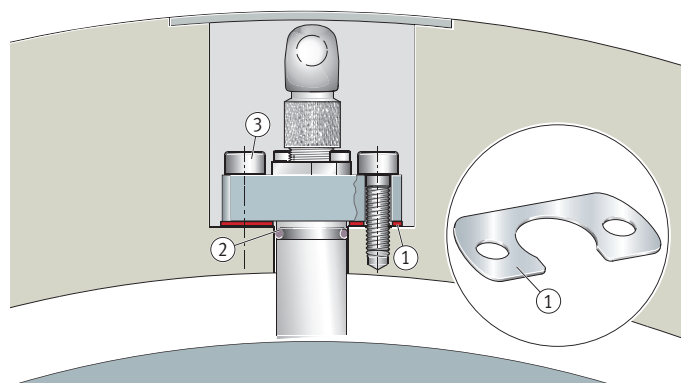
74 Messkopf einbauen
