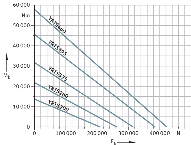
24 Statisches Grenzlastdiagramm für YRTS200 bis YRTS460
