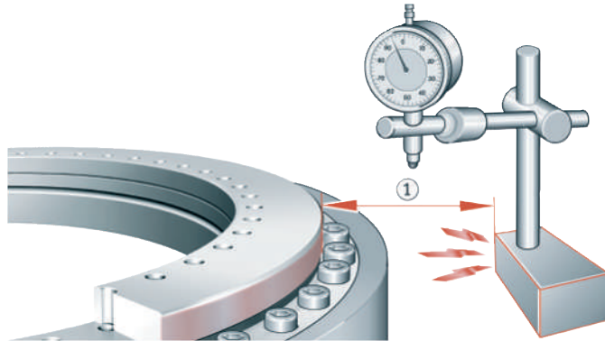
63 Mindestabstand magnetischer Messuhrstände zur Wellenscheibe
