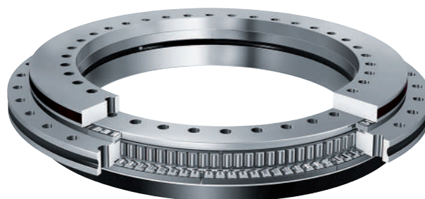
54 Axial-Radiallager mit magnetischer Maßverkörperung YRTCM, YRTSM
