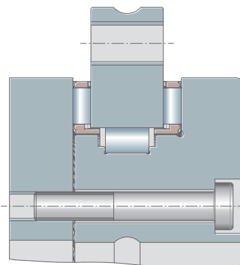
7 Angepasste Innenkonstruktion YRTA
