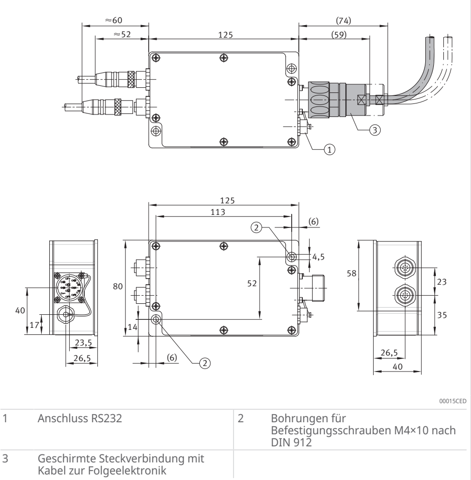
65 Anschlüsse und Abmaße der Auswertelektronik
