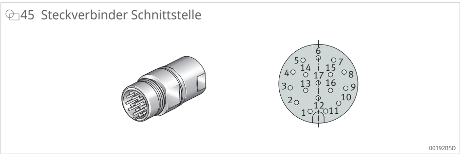
26 Anschlussbelegung
