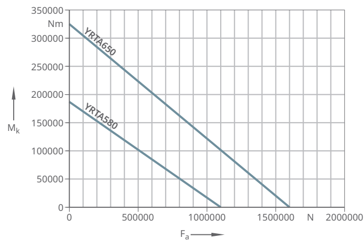
19 Statisches Grenzlastdiagramm für YRTA580 bis YRTA650
