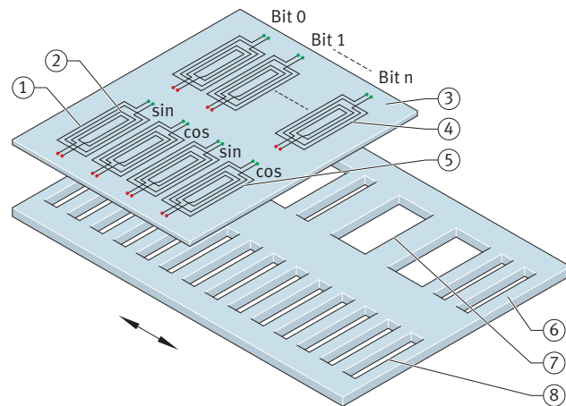
41 Wirkprinzip von induktiven, absoluten AMOSIN® Winkelmesssystemen
