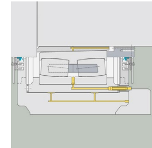
Sliding-Sleeve-Gehäuse
