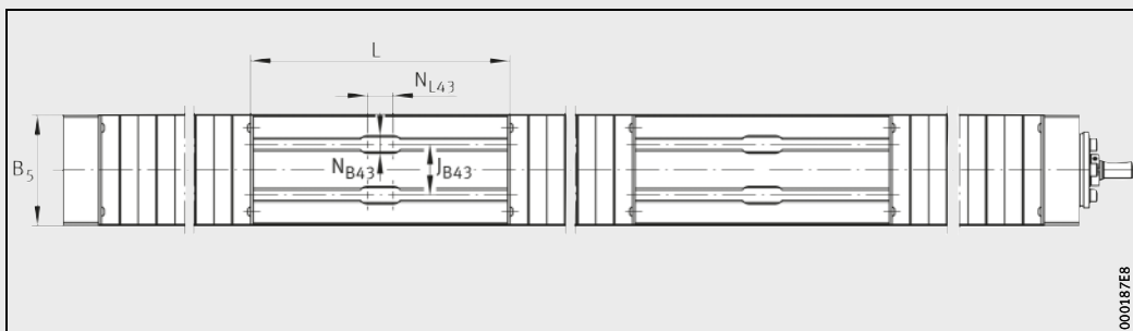
MKKUE20-200-KGT/5-N · Top view
