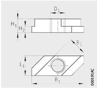
MU..-RHOMBUS · Rotatable T-nut
