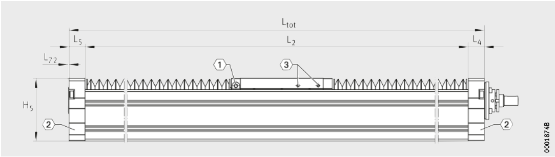
MKUSE25-200-KGT ①, ②, ③ 1)
