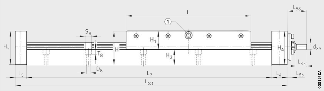
LTP, LTPG · Without bellows
