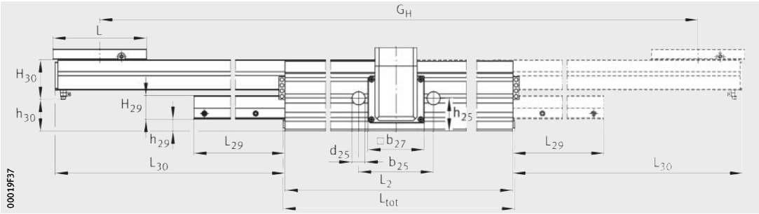
MTKUSE25-200-A-ZS/..-AO-N · Lateral view
