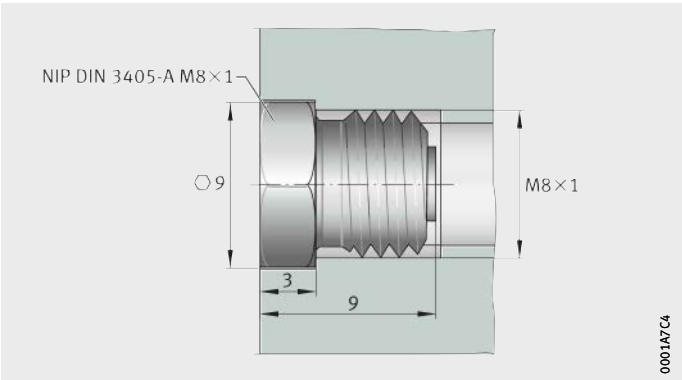
NIP DIN 3405-A M8x1
