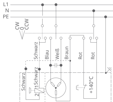
7 AC Einphasenwechselstrom : 120 V, 230 V
