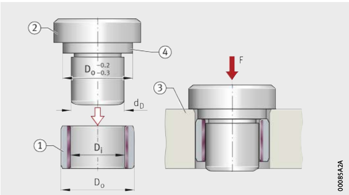
图 6 压装衬套沉入轴承座
