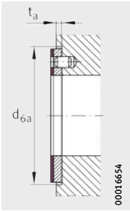
安装尺寸
