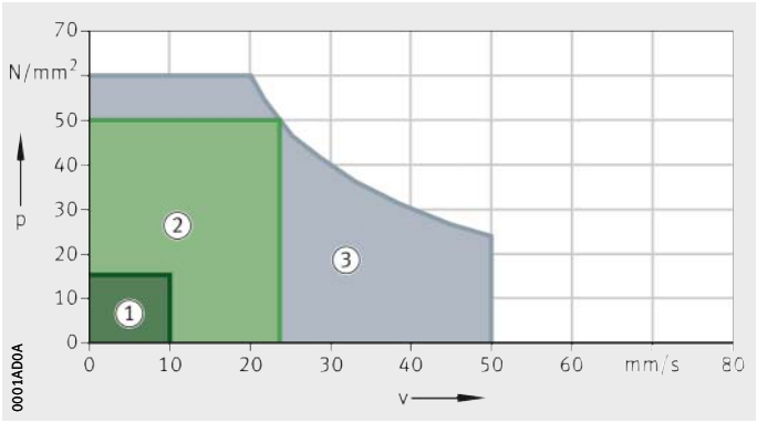
图 2 pv 图
