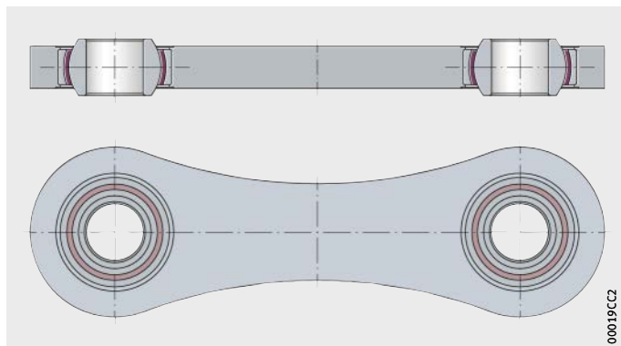
图 10 连杆
