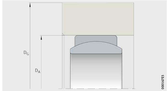
图 4 轴承座壁厚
