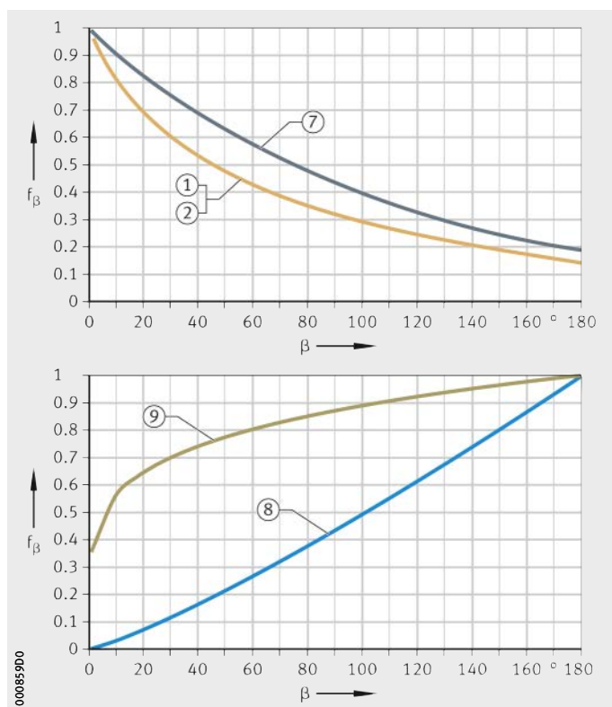
图 26 摆动角修正系数
