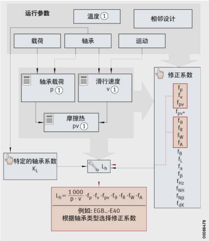
图 11 额定寿命计算过程
