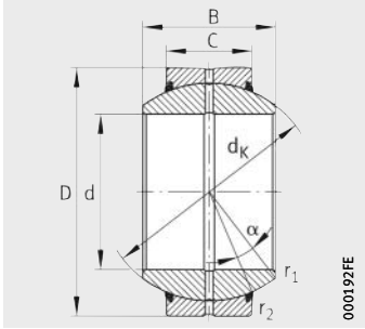
GE...FO-2TS 钢 / 钢
