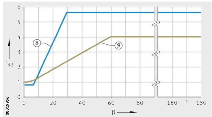
图 32 再润滑修正系数， 与摆动角 \beta 相关
