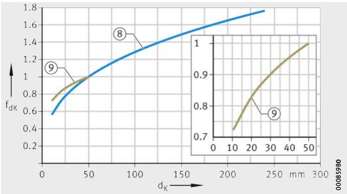
f_{dK} = 修正系数 d_K = 轴承球面直径 ⑧ 钢 / 钢 ⑨ 钢 / 青铜 图 22 球面直径修正系数
