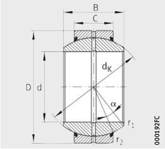
GE...FO-2RS 钢 / 钢
