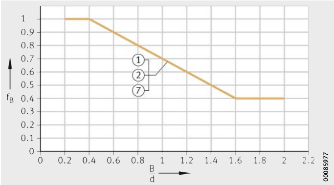
f_B = 修正系数 B = 轴承宽度 d = 轴承内径 ① ELGOGLIDE ② ELGOGLIDE-W11 ⑦ ELGOTEX 图 21 宽径比修正系数
