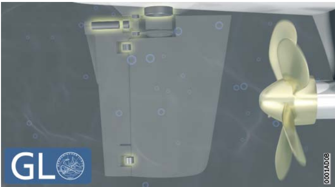
图 3 舵架轴承的应用
