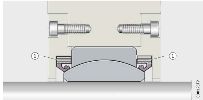
图 10 双组份密封
