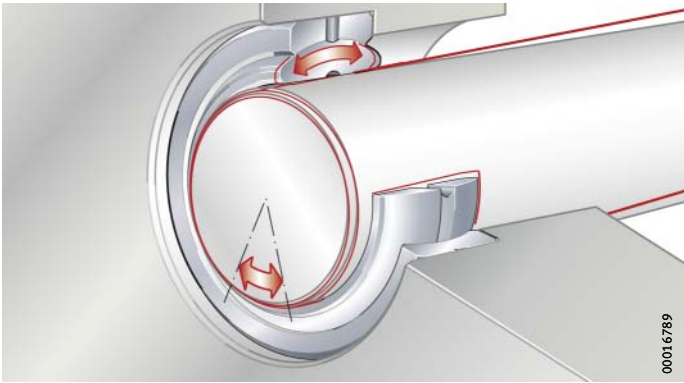
图 10 摆动和倾斜运动
