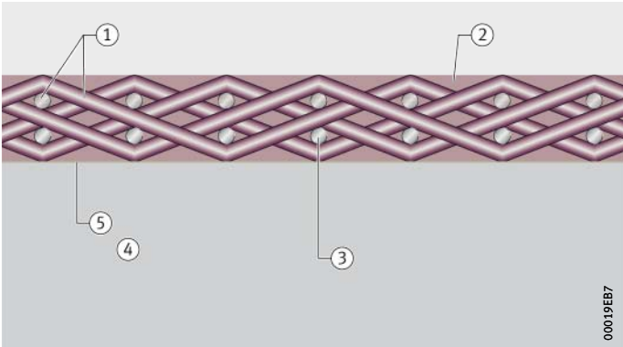
图 1 免维护衬套材料 ELGOGLIDE
