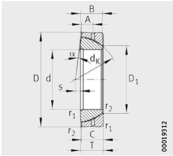
GE...-SX 钢 / 钢
