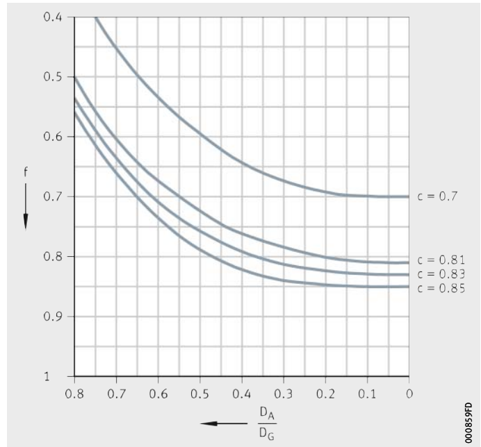
图 5 轴承座膨胀系数 f
