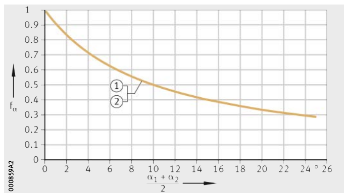
图 25 倾斜角修正系数
